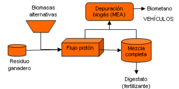
Diseño del proceso y de la planta de demostración
